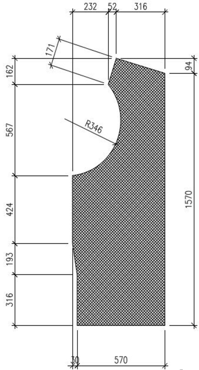
Pièce de base pour la borne "Taitorama" Les mesures sont donc en millimètres (oui, c'est précis...) Et oui, l'arrondi est chelou à comprendre avec ce plan...
